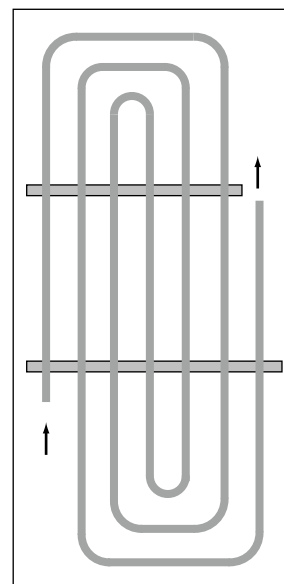
Draufsicht Wandheizungsregister
